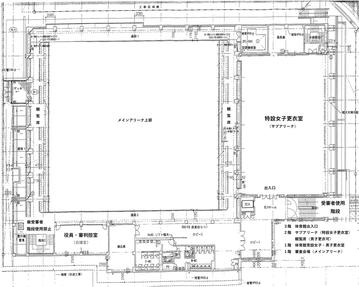
古曽部防災公園体育館 2階平面図
